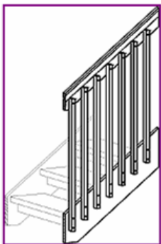
Kaide kylkikiinnityksellä (K) ja käsijohteella H1
